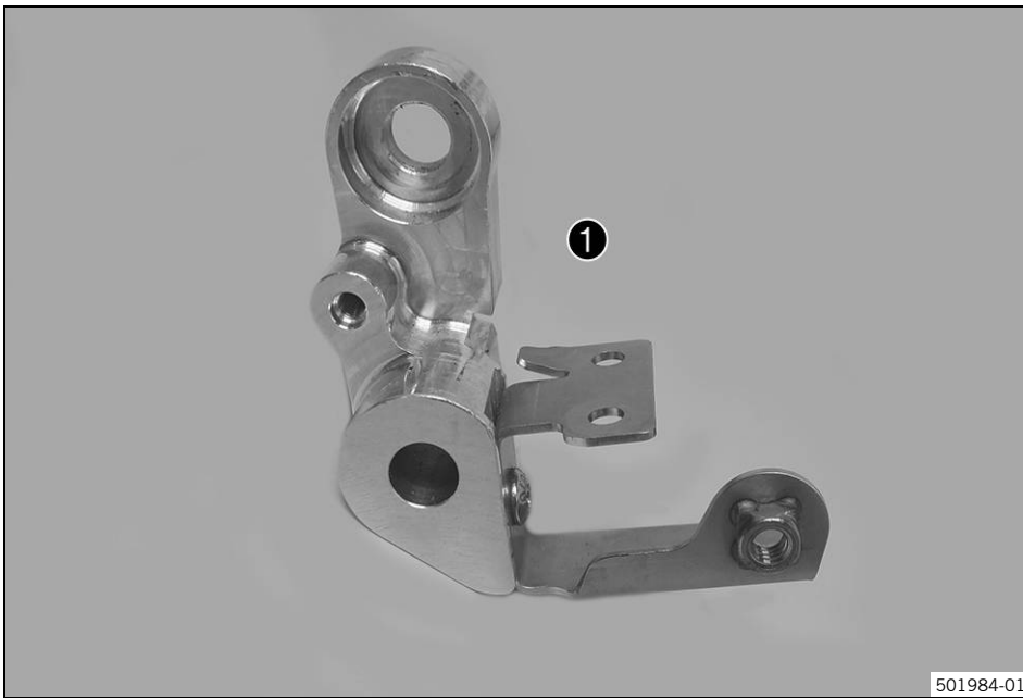
1x Kit di smontaggio cavalletto laterale ①
